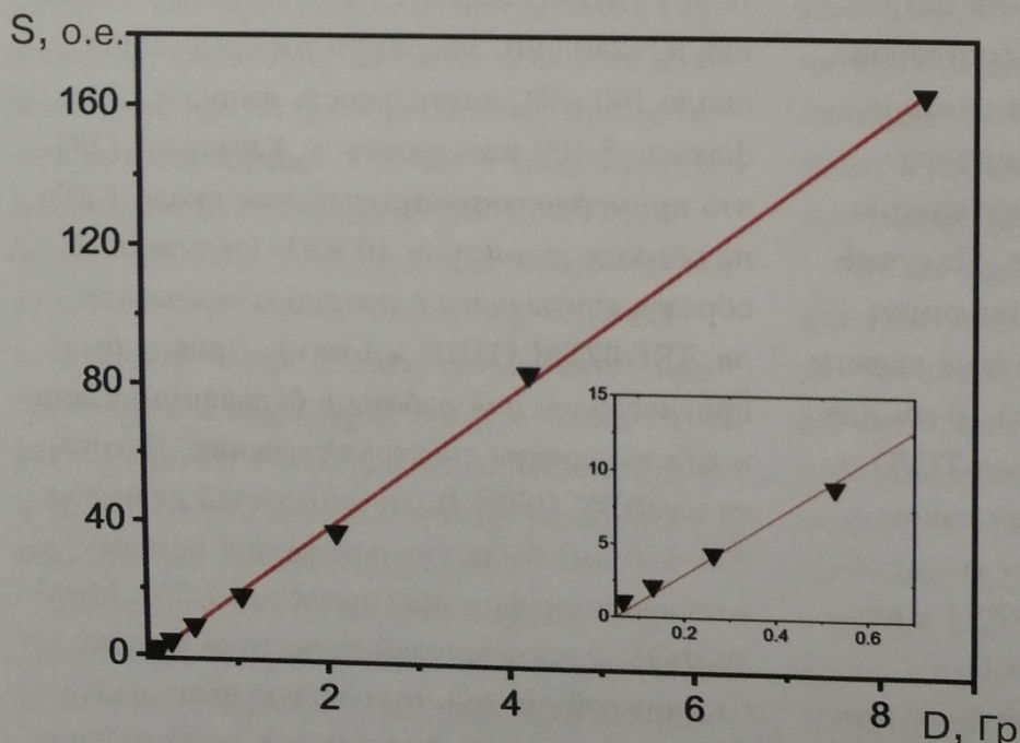
Рис. 1. Отклик детекторов ТЛД-580н на дозу радиации (площадь под рабочим пиком ТСЛ около 450 К). На врезке — начальный участок дозовой зависимости отклика.
