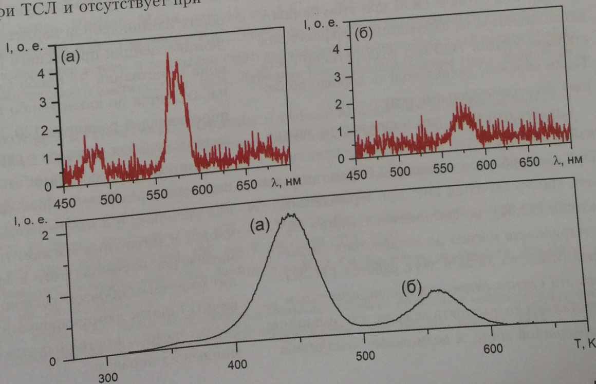
Рис.4. Кривая ТСЛ и спектры люминесценции (на вставках), соответствующие пикам ТСЛ, для детекторов ТЛД-580н на основе MgB_4O_7:Dy,Na .
