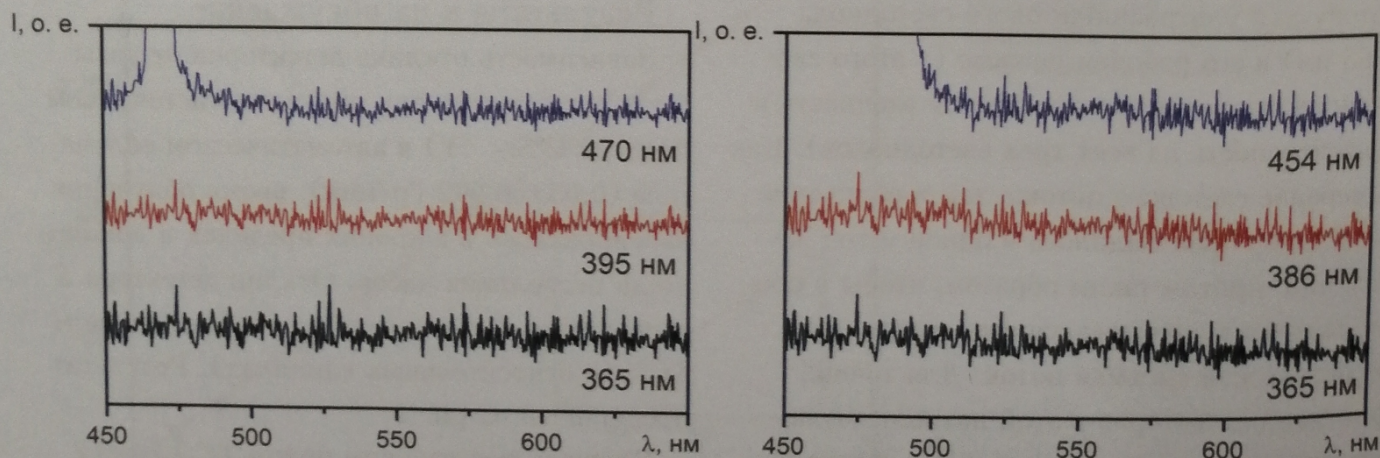
Рис.3. Отсутствие ОСЛ (под действием стимулирующего света 365, 395 и 470 нм) и ФЛ (при возбуждении светом 365, 386 и 454 нм) у детекторов на основе MgB_4O_7:Dy,Na .
